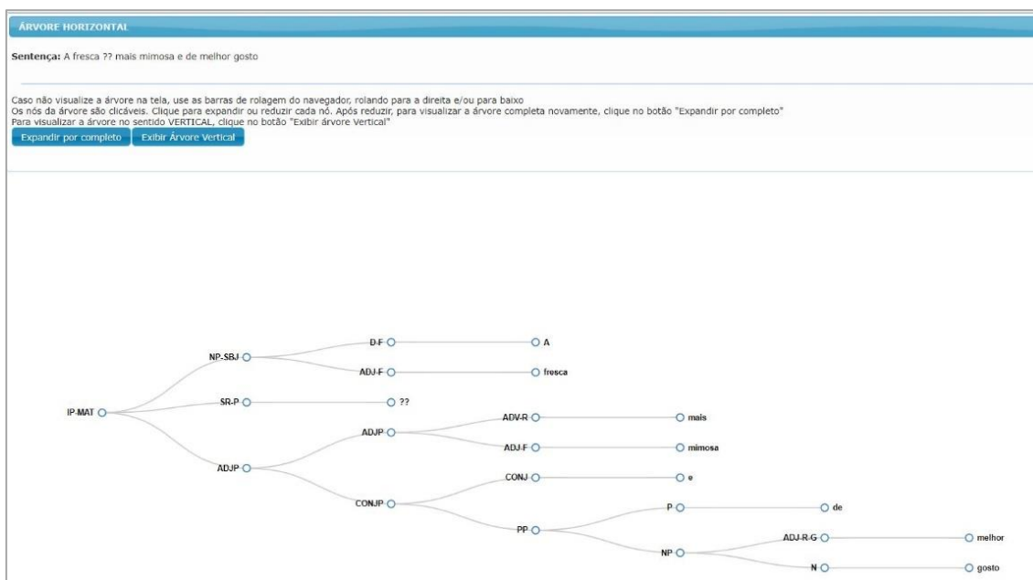
Figura 22 - Consulta ao Catálogo – Resultado de busca sintática (árvore sintagmática horizontal)
